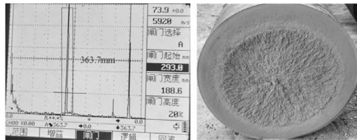
(a) 超声波探伤 (b) 断口形貌
