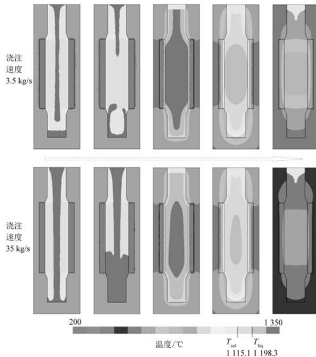
图7 不同浇注速度芯部重力流动充型及冷却阶段温度场数值模拟结果
