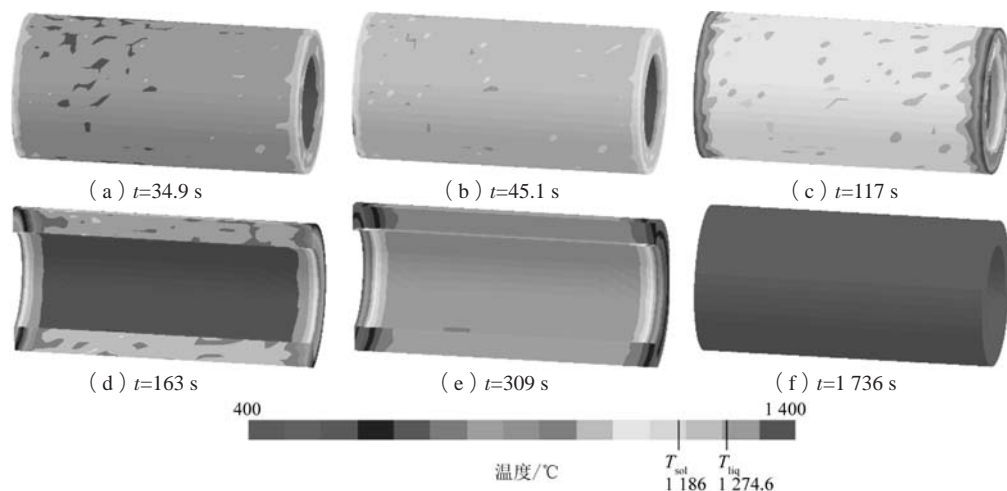
图4 900 r/min时外层离心冷却阶段温度场数值模拟结果
