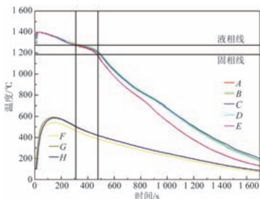
图5 900 r/min时外层和铸型离心过程各点温度变化
