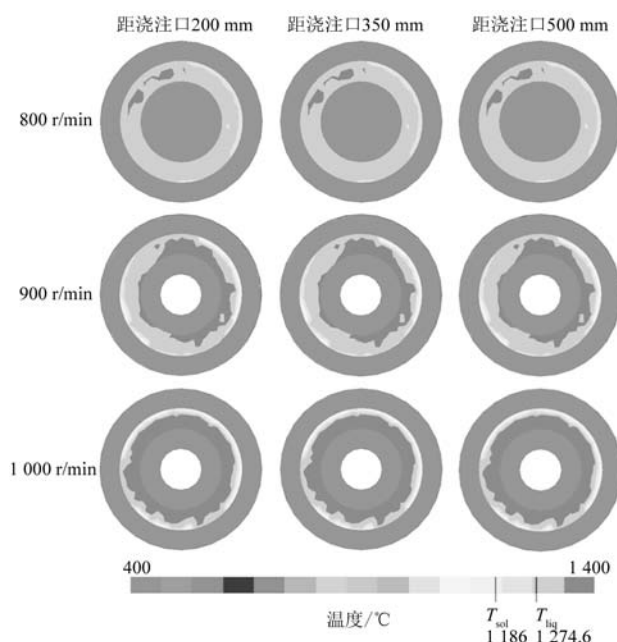
图6 不同转速外层横截面离心冷却阶段34.9 s温度场数值模拟结果
