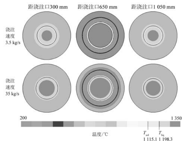
图8 不同浇注速度芯部横截面冷却阶段256 s温度场数值模拟结果
